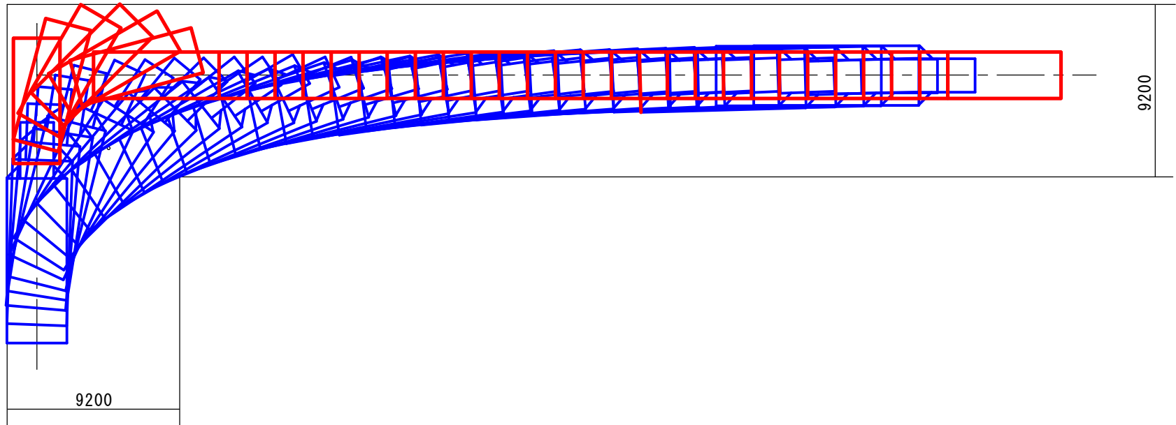
低床トレーラ軌跡図 (5800+5900)
